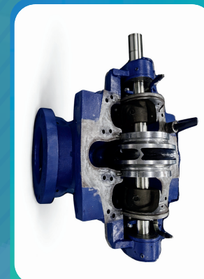
Bomba Bi-partida
